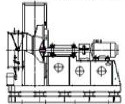
Исполнение 5 (на виброосновании)
