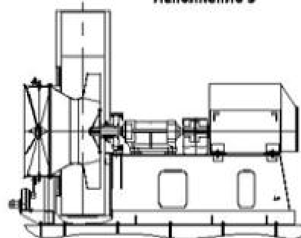
Исполнение 3
